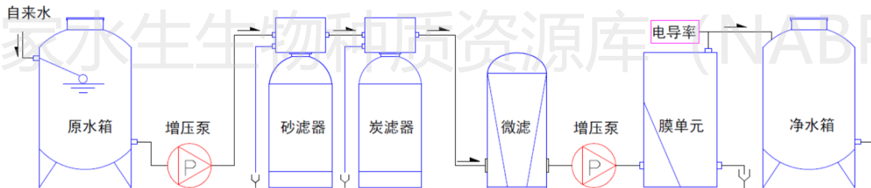
净水供水单元设备
