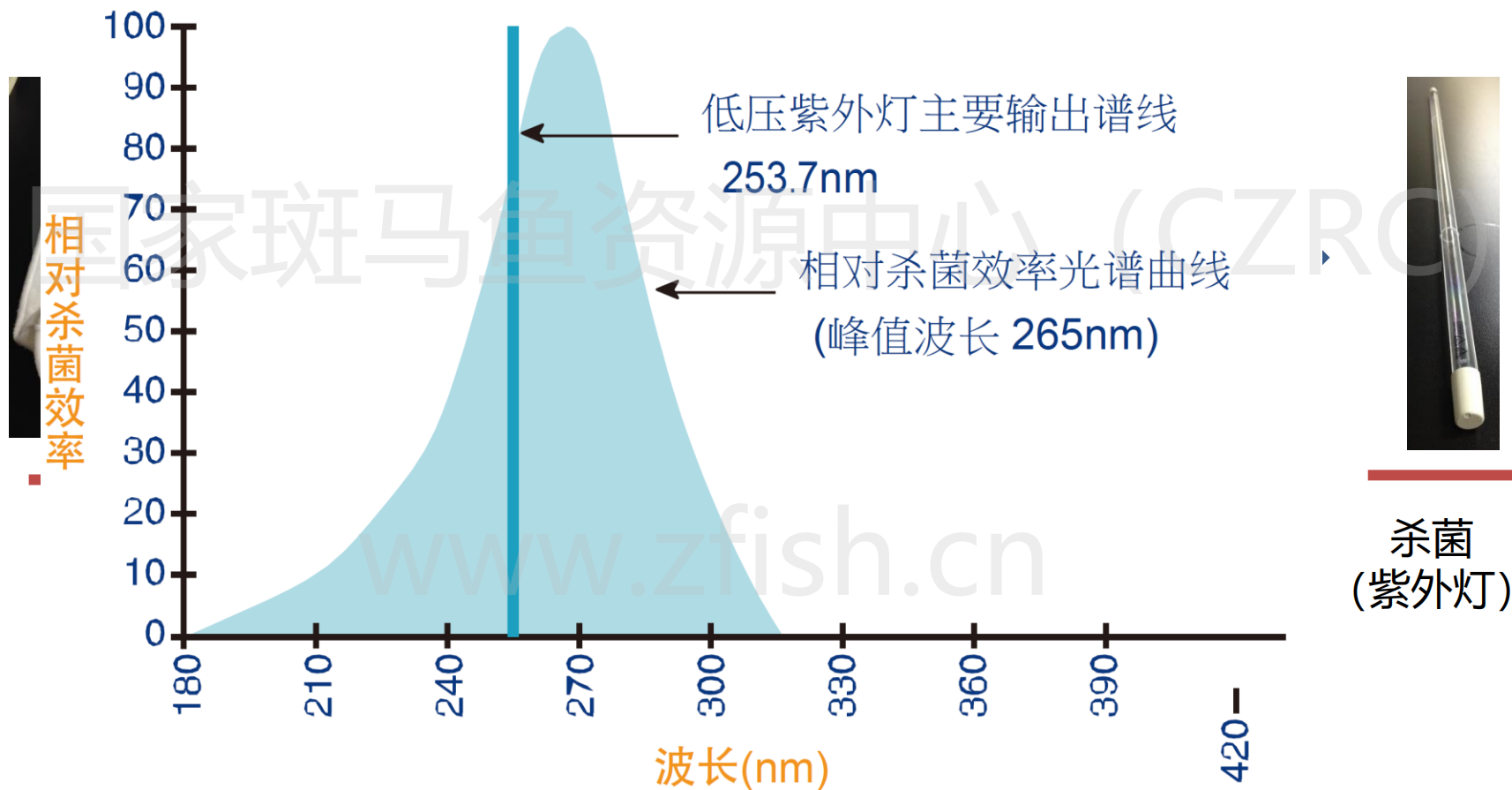
低压紫外灯杀菌效率图示
